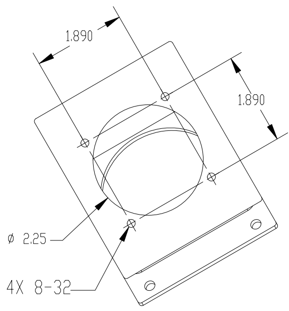
VIEW A-A
